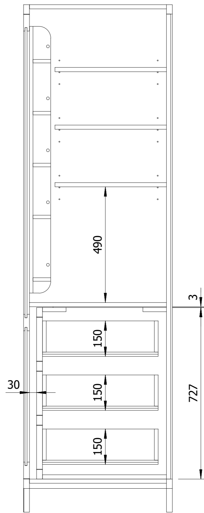
SECTION A-A
