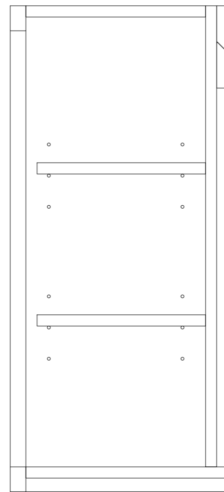
SECTION A-A
