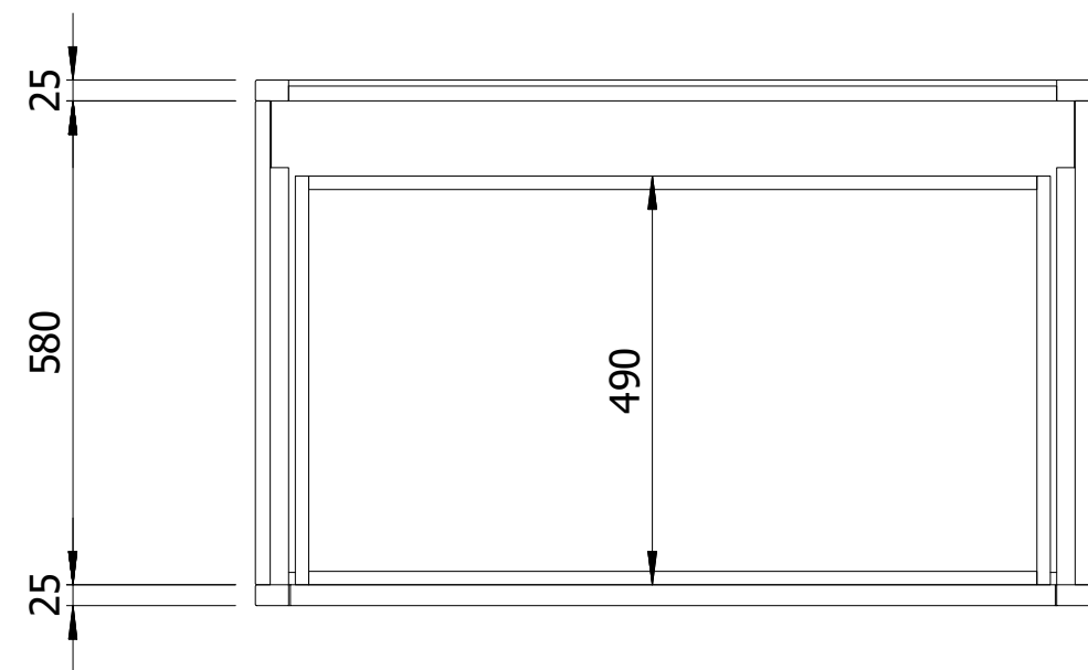
SECTION D-D
